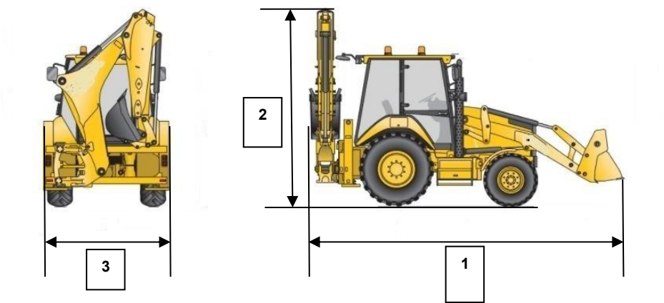
תמונה מס' 1 : שרטוט הצמ"ה
